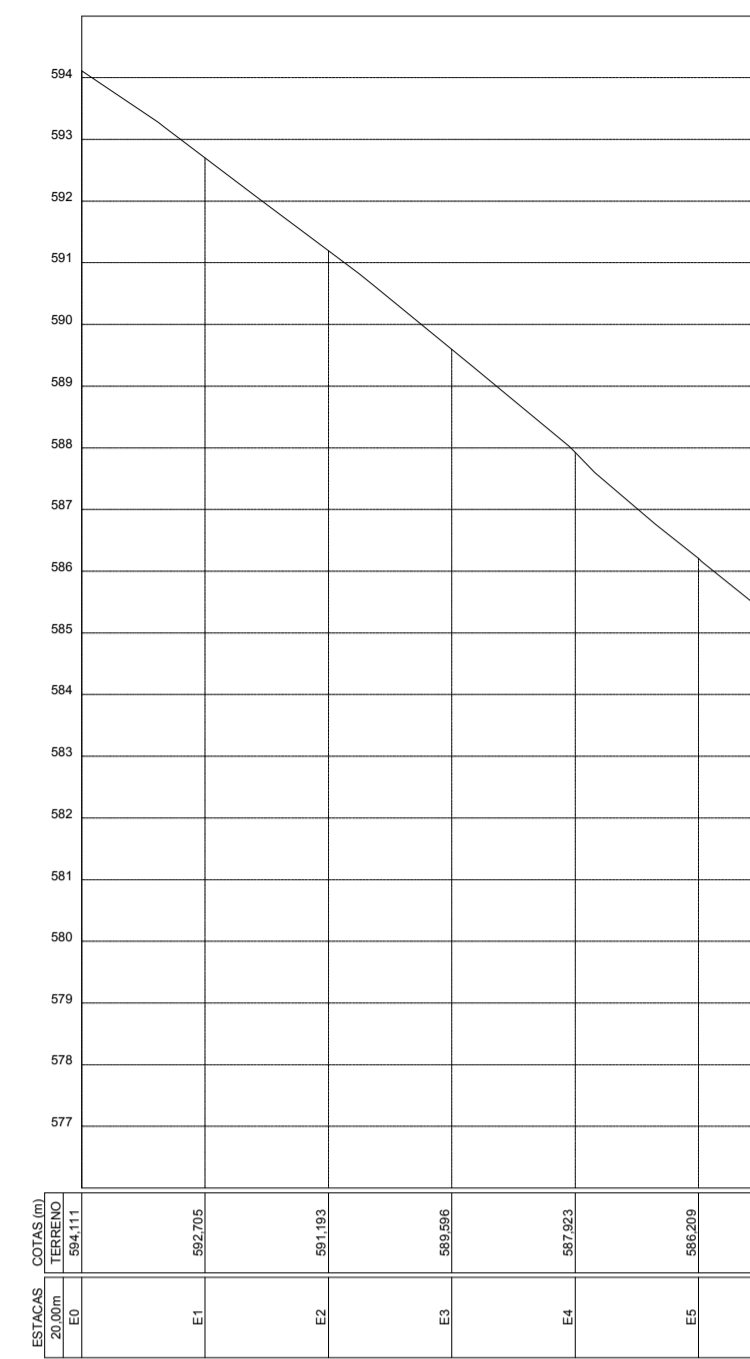
6 Perfil Longitudinal - Rua Oliveira Lima
