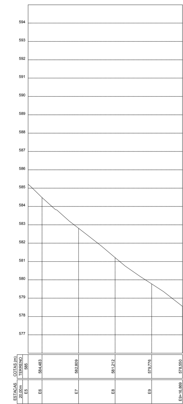
7 Perfil Longitudinal - Rua 7 de Setembro
