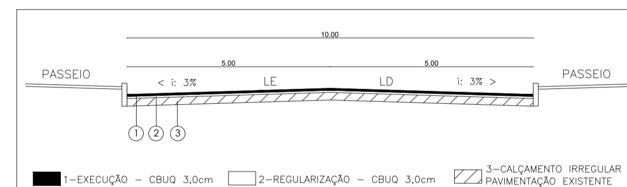
4 Perfil Transversal Rua Borges de Medeiros - Trecho 01
