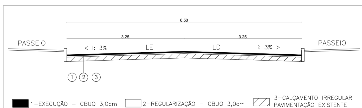
3 Perfil Transversal Rua 7 de Setembro
