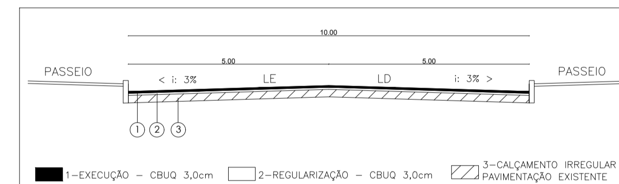
5 Perfil Transversal Rua Oliveira Lima
